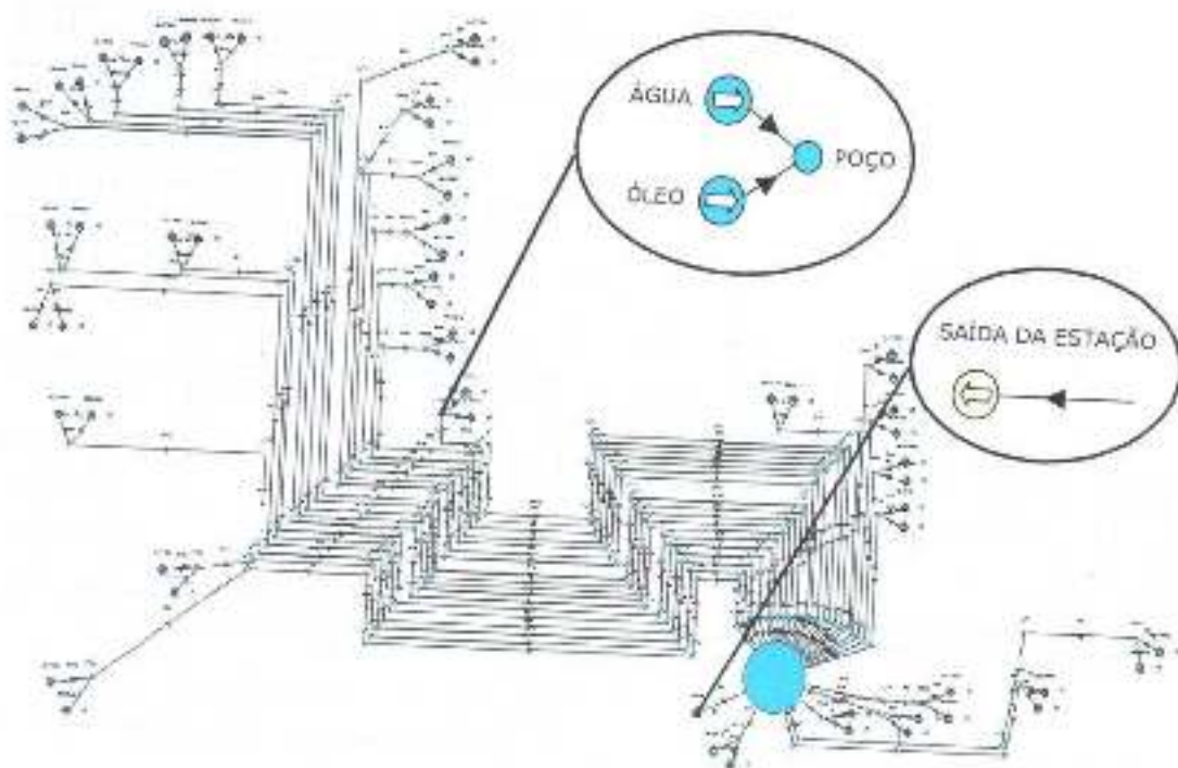
Figura 12: Malha de escoamento Poços — ETO.
