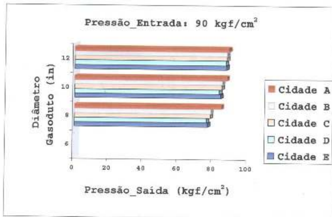
Figura 19: Resultados da simulação com pressão na entrada de 90 kgf/cm 2 .
