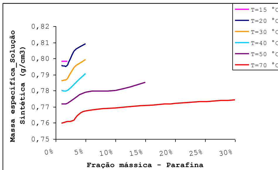
Figura 02 – Massa específica de soluções parafina/querosene em função da temperatura.
