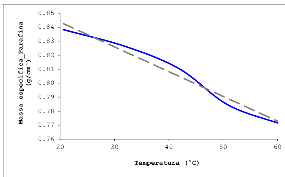
Figura 01 – Massa específica da parafina em função da temperatura.
