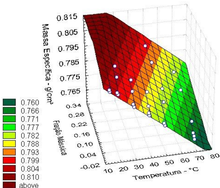
Figura 03 – Gráfico de superfície da massa específica em função da fração mássica e da temperatura.
