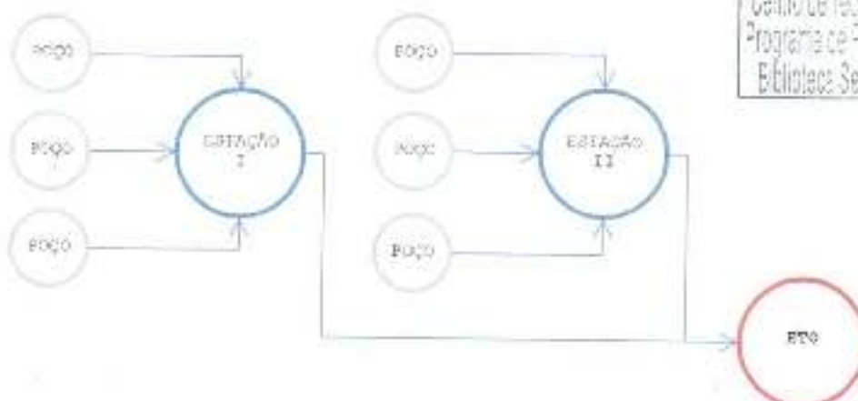
Figura 13: Esquema ilustrativo da malha de escoamento.
