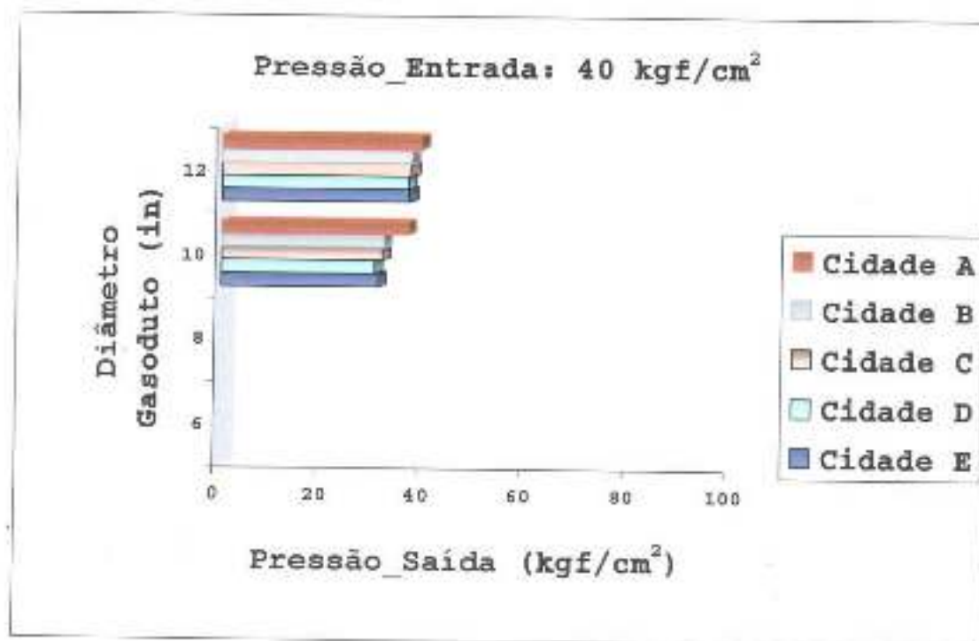
Figura 20: Resultados da simulação com pressão na entrada de 40 kgf/cm 2 .
