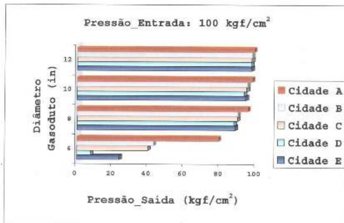
Figura 18: Resultados da simulação com pressão na entrada de 100 kgf/cm 2 .
