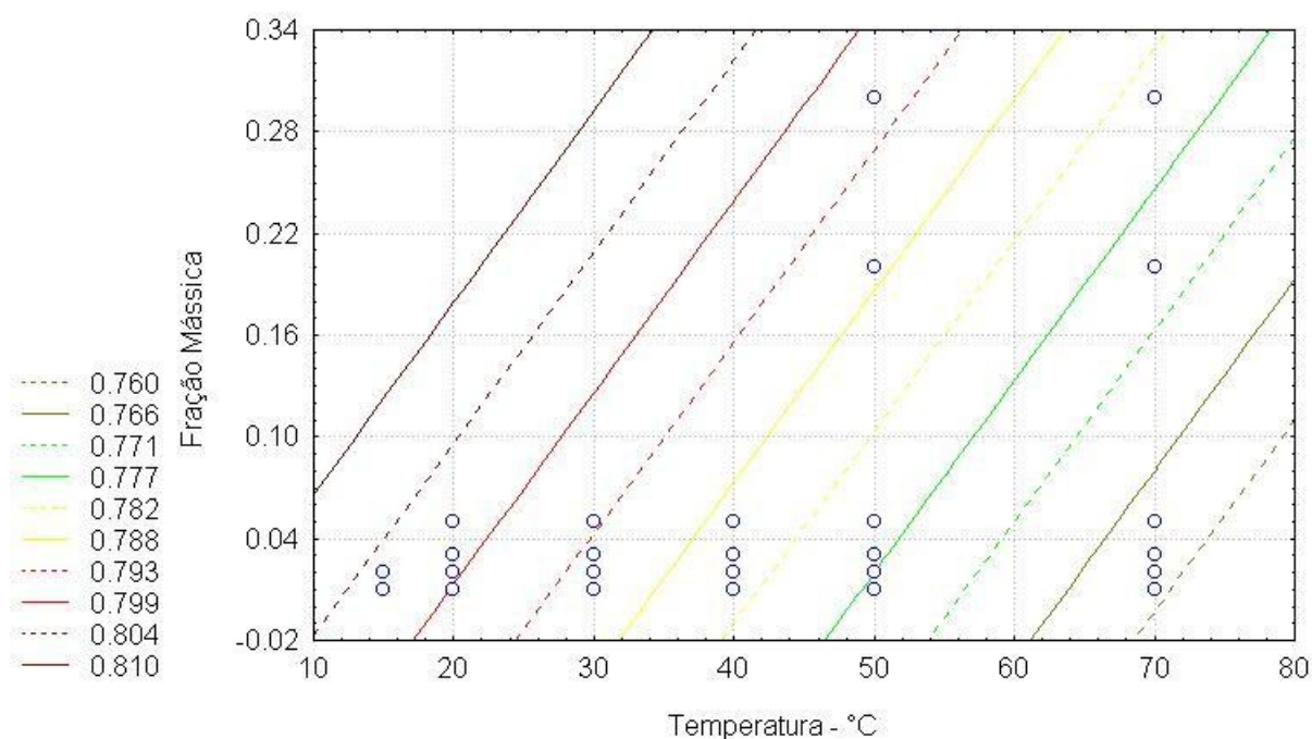
Figura 04 – Curvas de massa específica em função da fração mássica e da temperatura.
