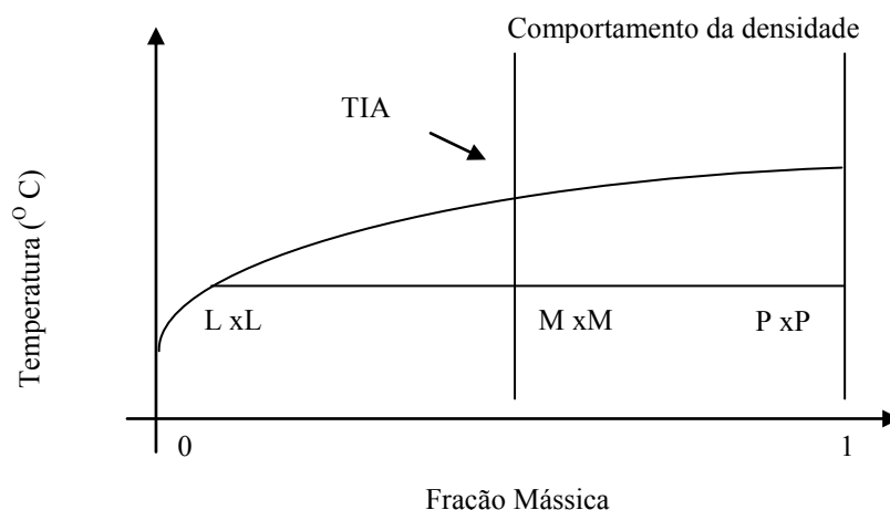
Figura 06 – Diagrama de Fases.
