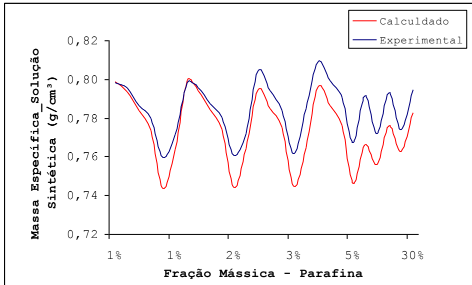
Figura 05 – Curvas de massa específica em função da fração mássica e da temperatura.
