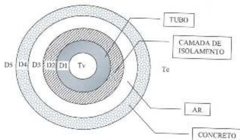
Figura 06: Tubulação isolada, revestida, enterrada e com injeção de vapor.
